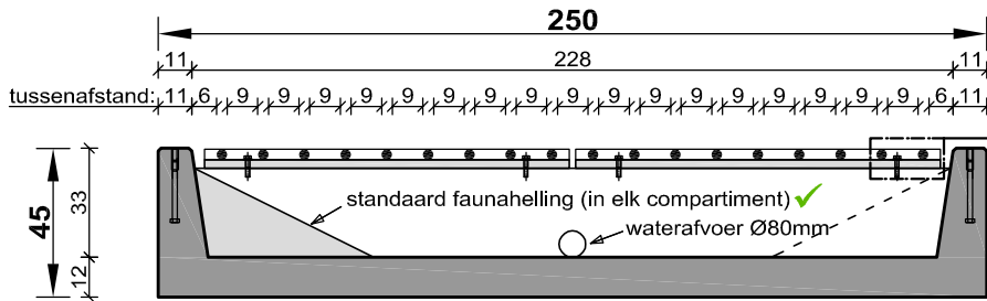
dwarsdoorsnede AA
